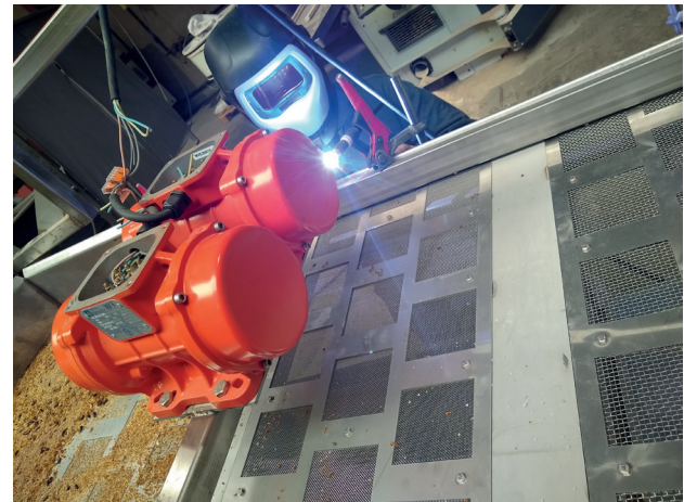
Meelwormzeefmachine van Tor Royal in samenwerking met Vermeulen Construct
